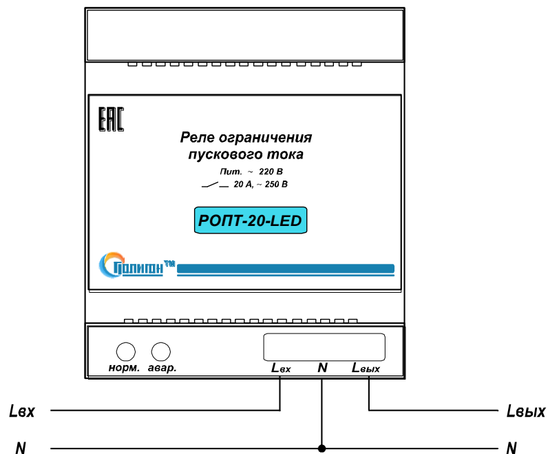
Рис.1. Типовая схема подключения РОПТ-20-LED.
